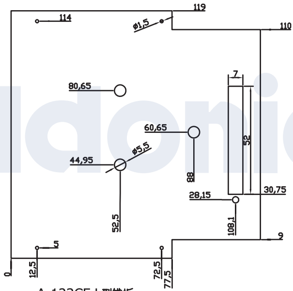
A-123CF L型鐵板
